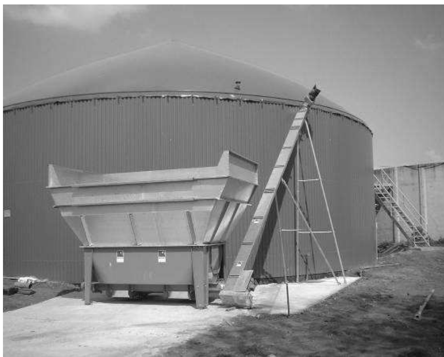
Rysunek 8. Przykład zbiornika wstępnego na substraty stałe z systemem dozowania (źródło: WWW.ieo.pl)
