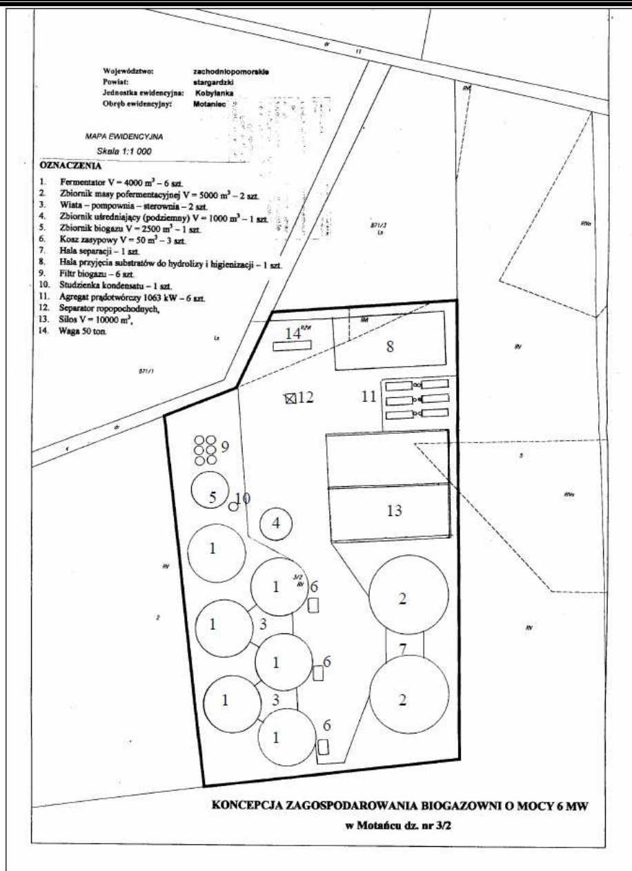
Rysunek 5. Schematyczne usytuowanie rozmieszczenia elementów przedsiębiorstwa
