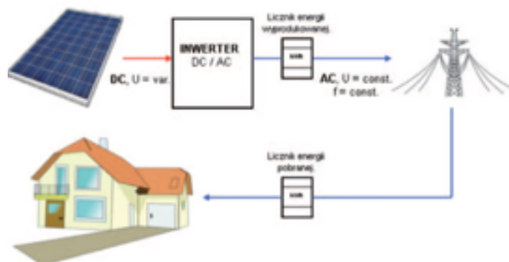
Rysunek 25. Schemat instalacji ON-GRID 130 (oznaczenia: DC- prąd stały, AC-prąd przemienny, U- napięcie, f-częstotliwość, var.-zmiennie, const.- stałe)
