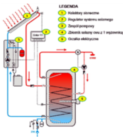
Rysunek 18. Schemat typowej instalacji słonecznej do podgrzewania ciepłej wody użytkowej 116
