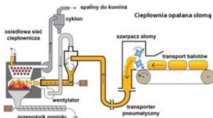
Rysunek 20. Schemat kotłowni na słomę 121
