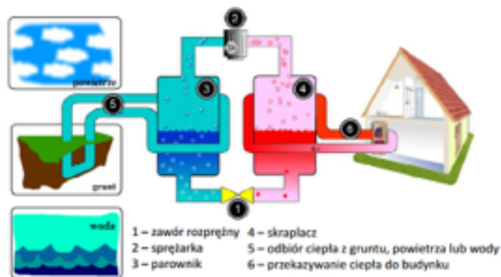
Rysunek 17. Zasada działania pompy ciepła 113
