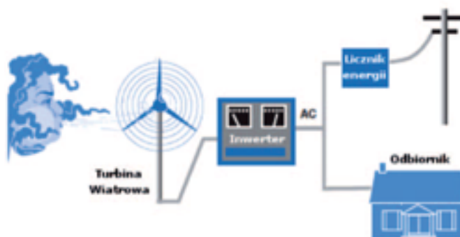
Rysunek 24. System zasilania gospodarstwa domowego zintegrowany z siecią energetyczną 127 .
