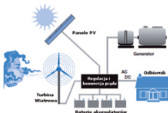
Rysunek 23. Automatyczny (wyspowy) system zasilania gospodarstwa domowego 126
