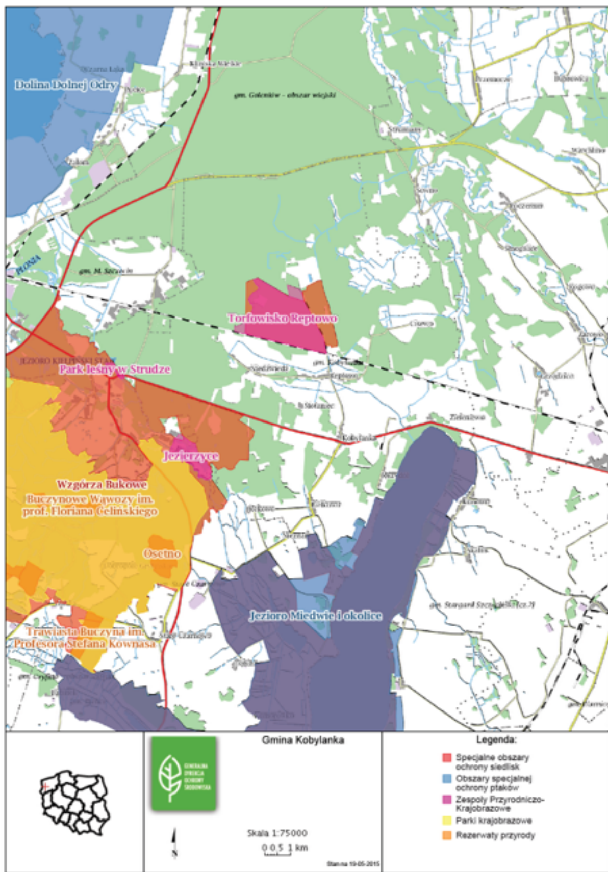
Rysunek 2. Lokalizacja obszarów chronionych w gminie Kobylanka. 34
