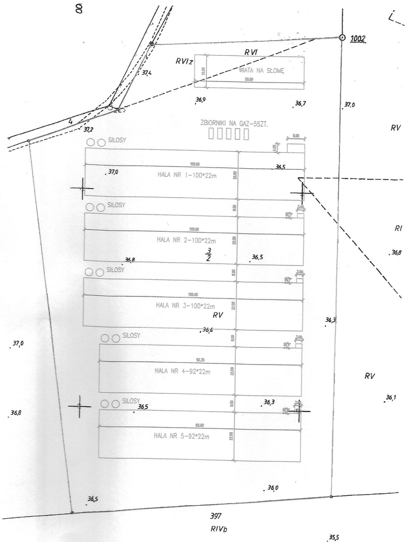
Plan fermy drobiu w Motańcu dz. 3/2 Rys. 3
